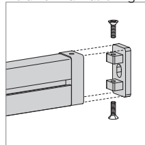
Particolare aggancio a parete
